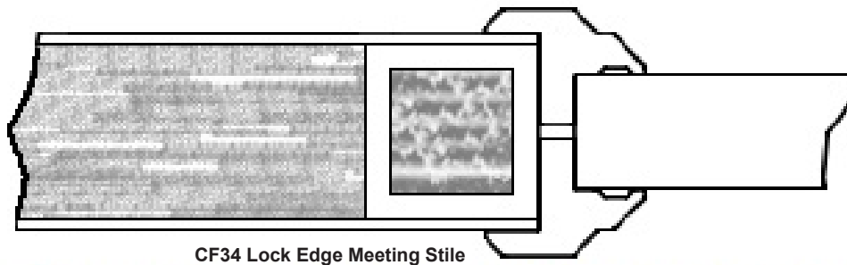
CF34 Lock Edge Meeting Stile
